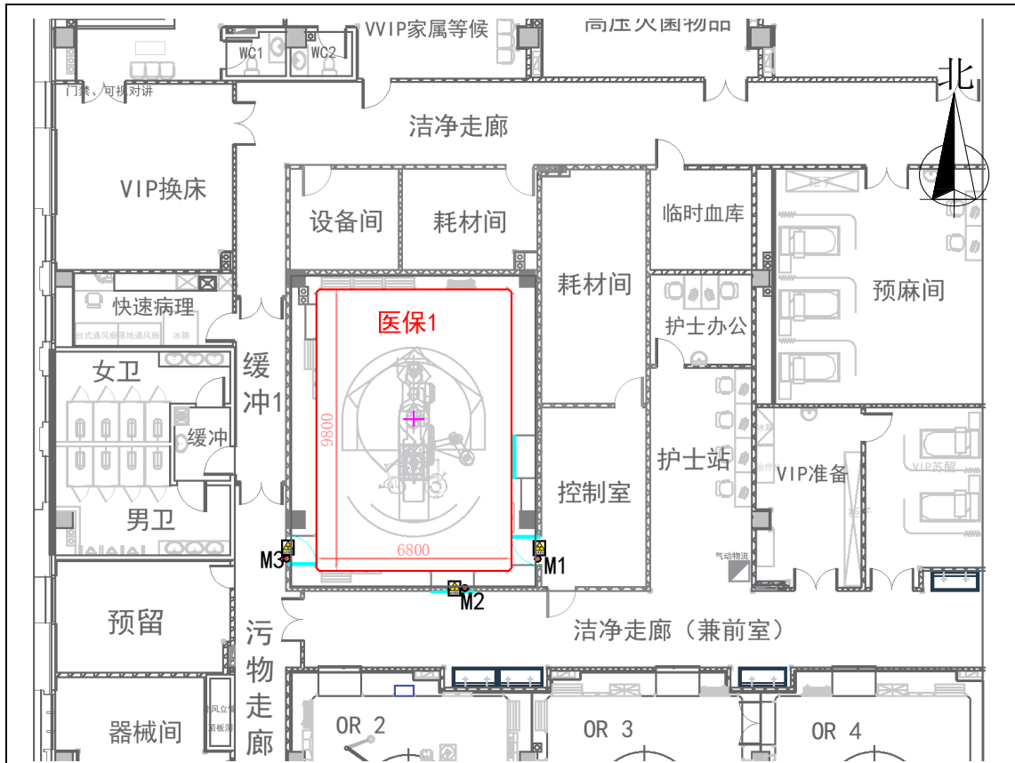
图 7-2 医保 1 室四周毗邻关系图
