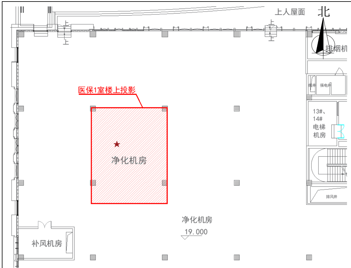
图 12-2 医保 1 室（楼上）自行检测点位图（标注★为检测位置）
