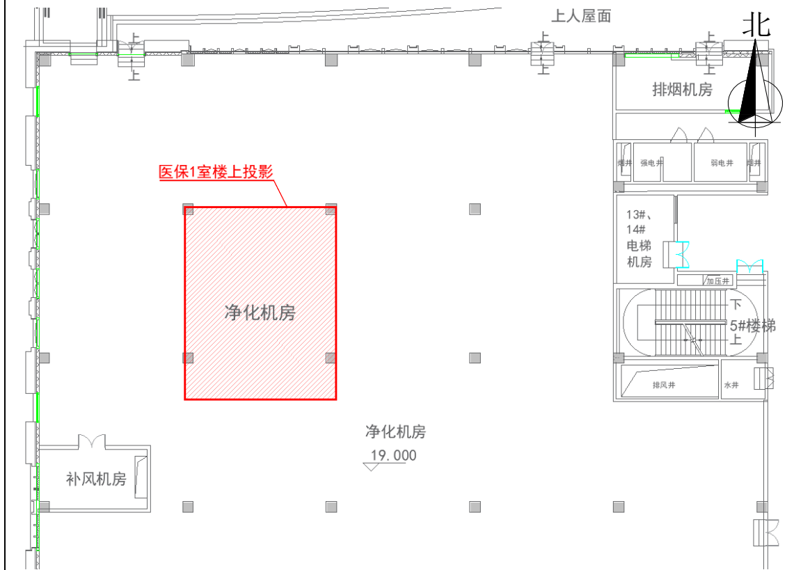
图 7-3 干保医技综合楼 5 层平面布局示意图（医保 1 室上方）
