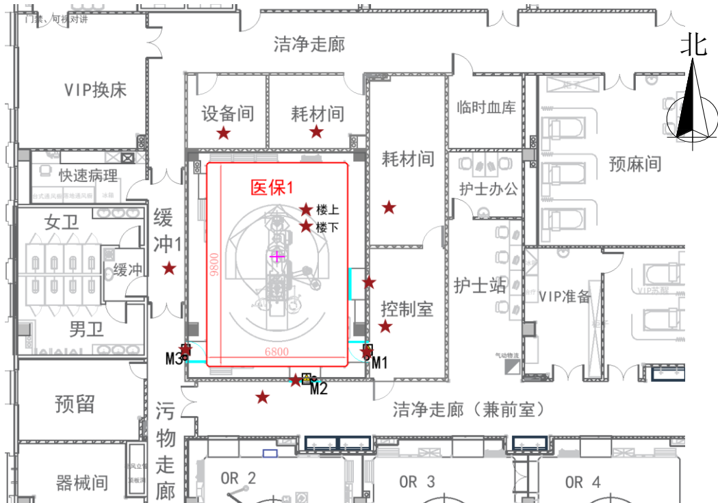
图 12-1 医保 1 室周围自行检测点位图 (标注★为检测位置)
