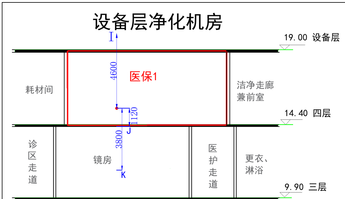
图 11-3 医保 1 室楼上、楼下南北向剖面图
